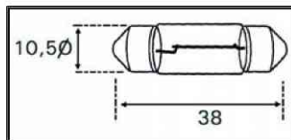
SV8,5
