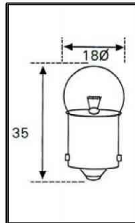
BA-15s
