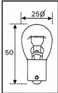
BA15s
